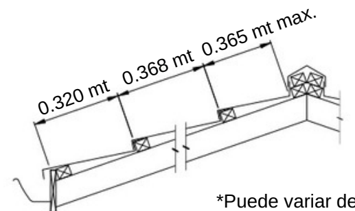
Sección del Solape
